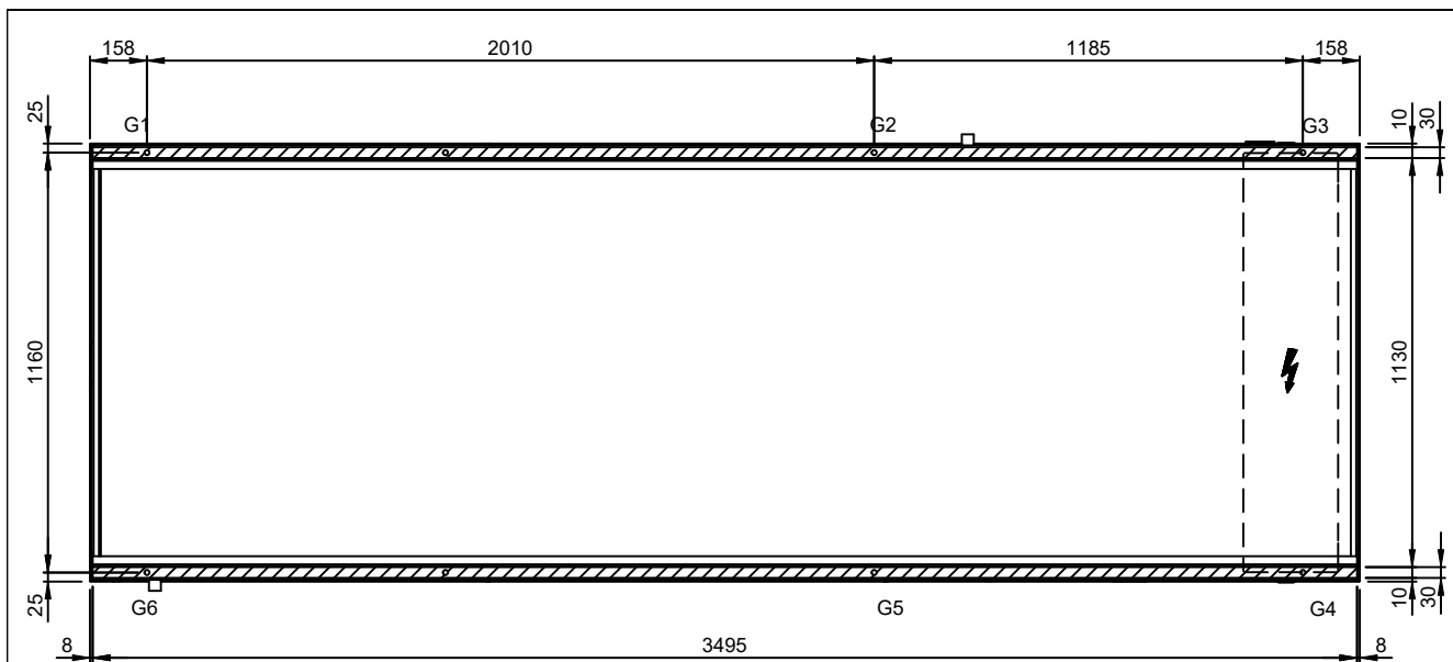
PODSTAWA URZĄDZENIA \ FOOTPRINT
