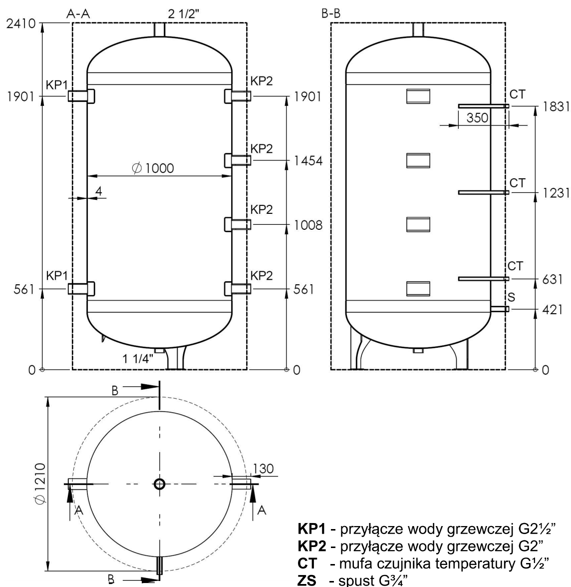
Rys. Zbiornik buforowy DIS 1500
