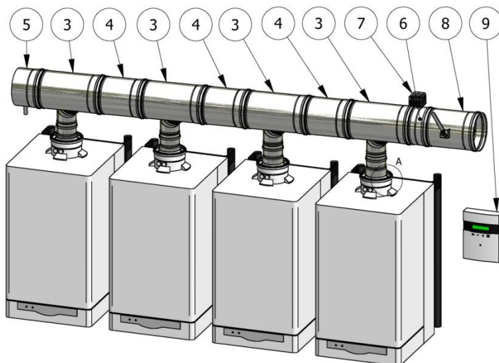
Schemat podłączenia elementów spalinowych do 4 kotłów Vitodens 200-W typ B2HA
