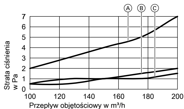
Straty ciśnienia na przejściu z 2 króćcami przyłączeniowymi rozdzielacza
