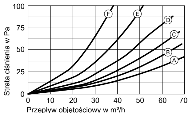
Prostokątna obudowa przepustu powietrza R75 L z 1 pokrywą zamykającą i kratką podłogową lub ścienną, powietrze usuwane
