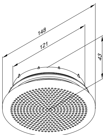
Okrągła dekoracyjna kratka powietrza wywiewnego
