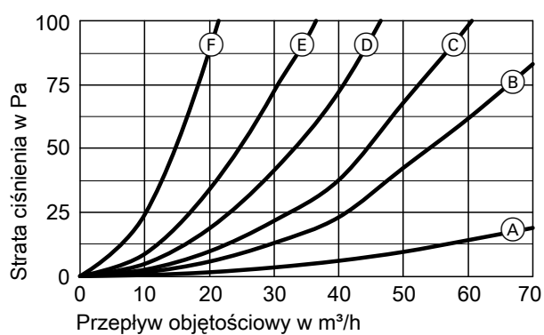
Prostokątna obudowa przepustu powietrza F50 S z kratką podłogową i ścienną, powietrze dolotowe
