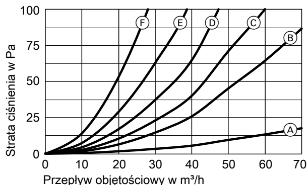
Prostokątna obudowa przepustu powietrza R75 L z 1 pokrywą zamykającą i kratką podłogową lub ścienną, powietrze dolotowe
