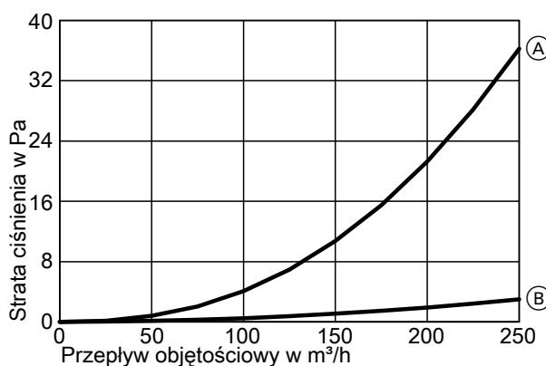
Straty ciśnienia
