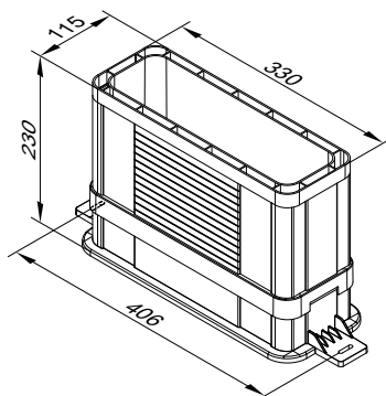
Prostokątna nakładka montażowa 230 mm
