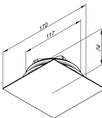
Kwadratowy anemostat powietrza nawiewnego/wywiewnego Vitoair
