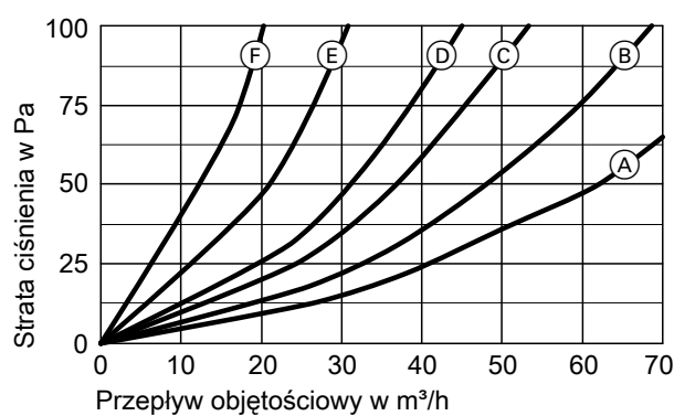
Prostokątna obudowa przepustu powietrza F50 S z kratką podłogową i ścienną, powietrze usuwane
