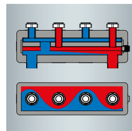
Zintegrowane sprzęgło hydrauliczne (typy: GMA411, GMA521, GMA531)
