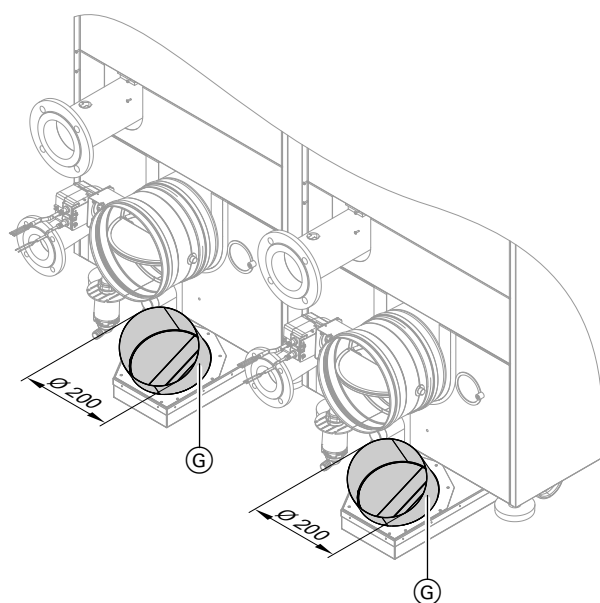
Skrzynka z przewodem powietrza dolotowego kotła Vitocrossal, typ CI3 480
