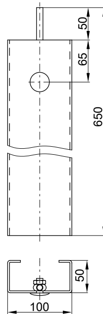
Wymiar systemowy 250
