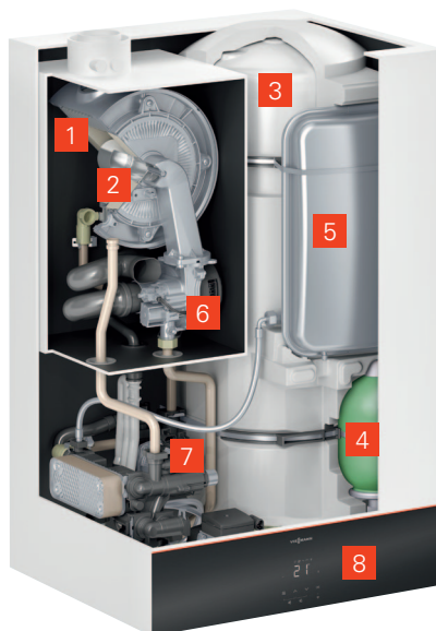
VITODENS 111-W (Typ B1LF)
