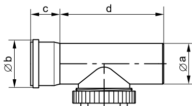
Kształtka rewizyjna (prosta)
