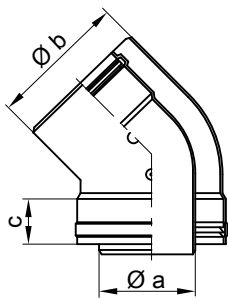
Kolanko do ściany zewnętrznej 45°
