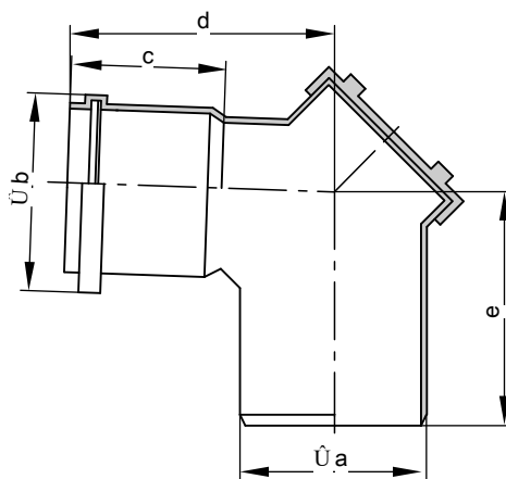
Kolano rewizyjne
