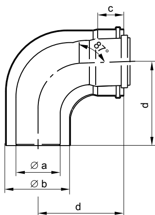
Wymiar systemowy Ø 110 mm
