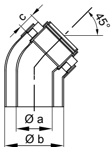
Wymiary systemowe Ø 60 i 80 mm
