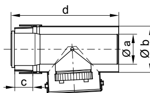
Wymiary systemowe Ø 60 mm
