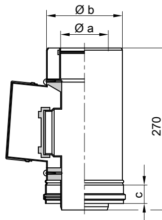
Kształtka rewizyjna do ściany zewnętrznej
