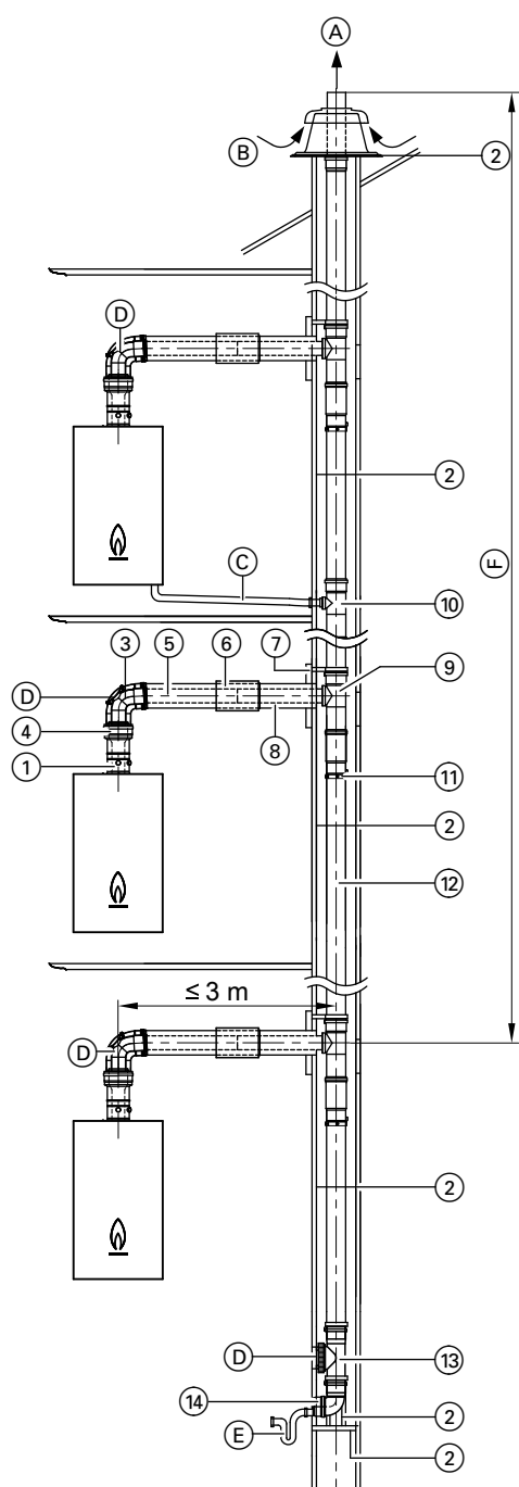
1 kotioł grzewczy na piętro
