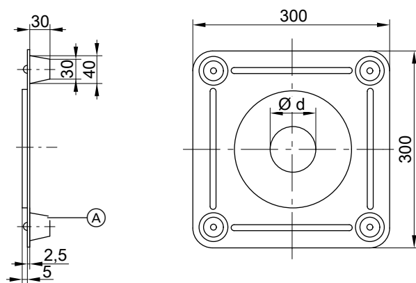
Oslona nawiewu
