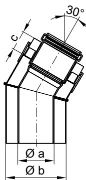
Wymiary systemowe Ø 60 i 80 mm
