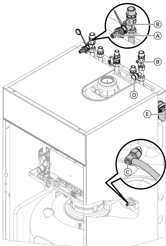
Rys. 28 Urządzenie z przyłączami skierowanymi do góry
