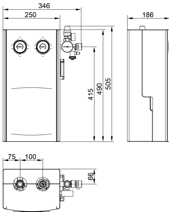
Zestaw pompowy Solar-Divicon
