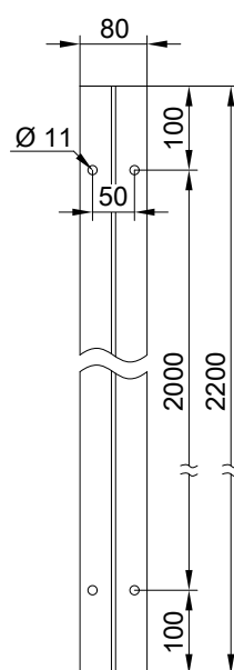
Wymiar otworów ramienia podstawy
