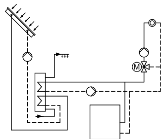
Instalacja z dwusystemowym, pojemnościowym podgrzewaczem cwu
